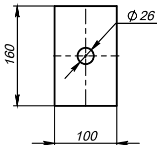
Поз.2 (Накладка)
