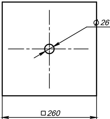
Поз.3 (Плита опорная)
